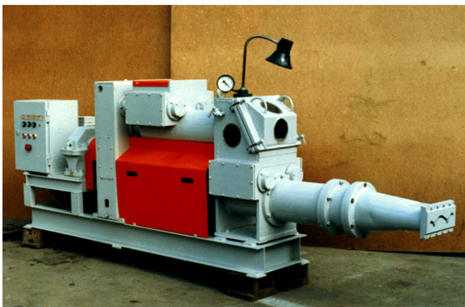
Вакуум-Пресс ВП-200 с насадкой для вытягивания черепицы
